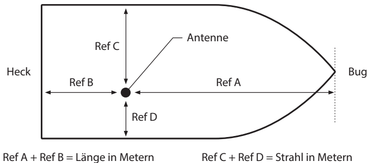
Abbildung 35 GNSS-Antennenposition
