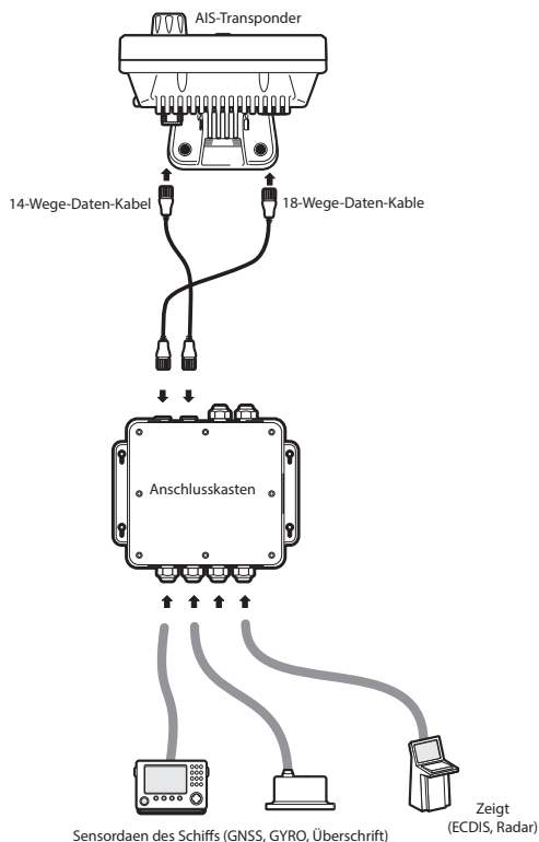
Abbildung 34 Anschluss externer Geräte
