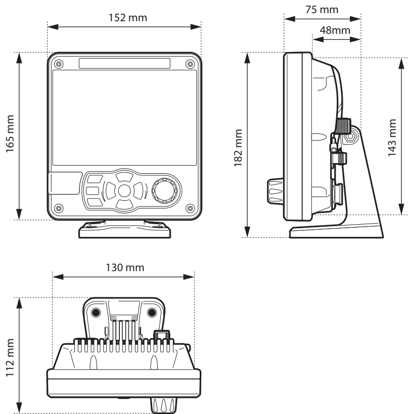
Abbildung 30 Abmessungen des Transponders
