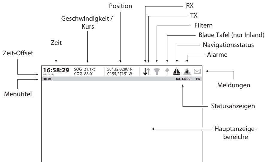
Abbildung 21 Display-Layout
