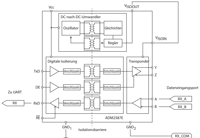
Abbildung 28 Schema des Eingangsports
