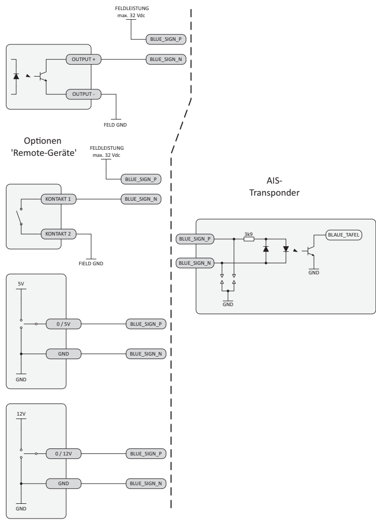
Abbildung 27 Anschlussoptionen für die 'Blaue Tafel'-Schnittstelle
