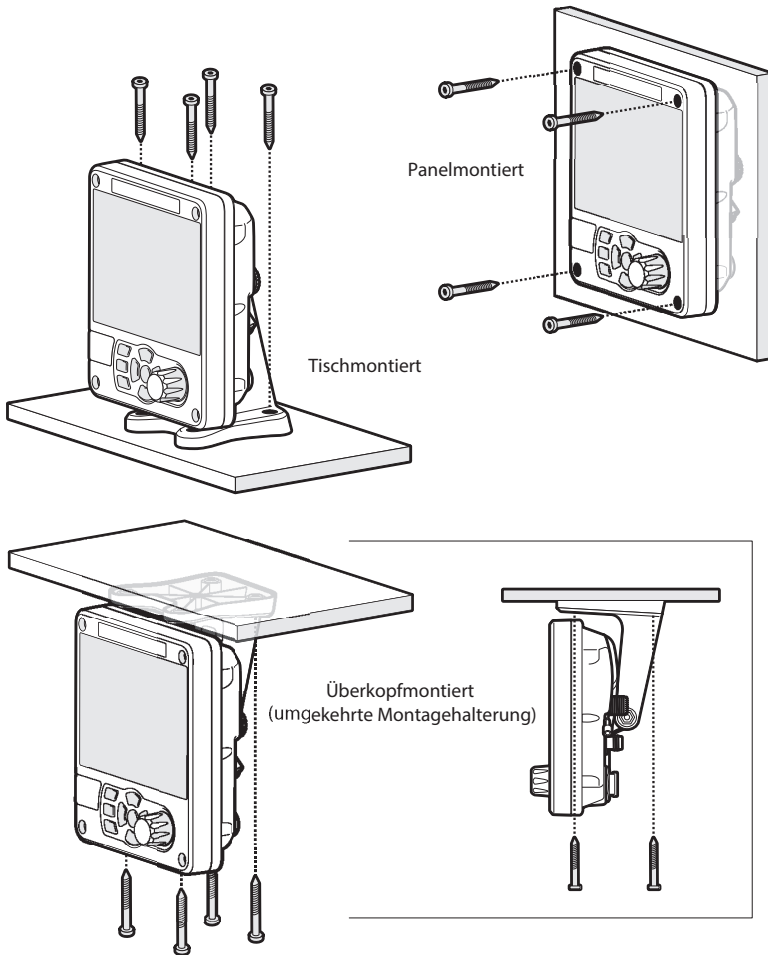
Abbildung 4 Montage des Transponders
