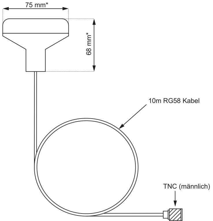
Abbildung 31 GNSS-Antenne
